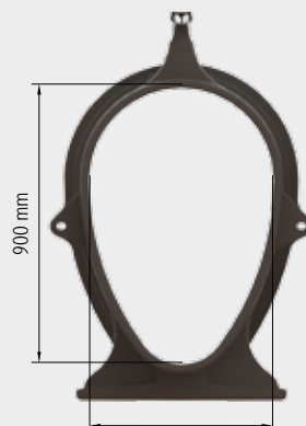
600 mm tojásszelvény Qmax 900
