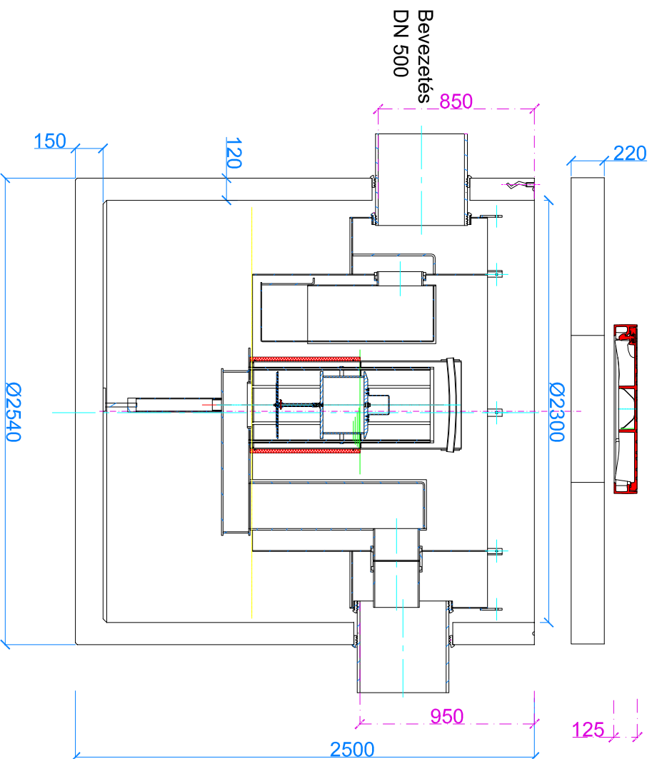
A metszet
