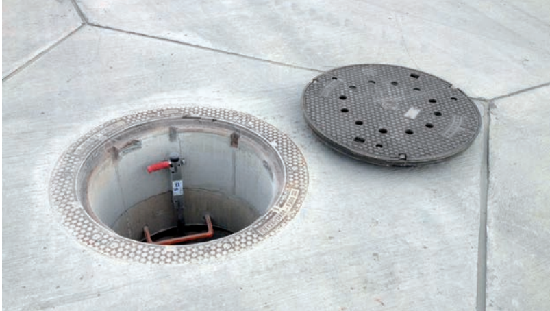
Gussabdeckung mit Schraubvorreiber-Verschlüssen Belastungsklasse F900, lichte Weite 800 mm
