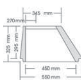
K11 / kúp elem Súly: 51 kg
