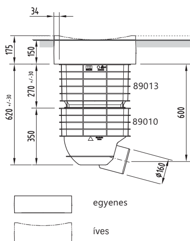
500 x 500 rövid akna
