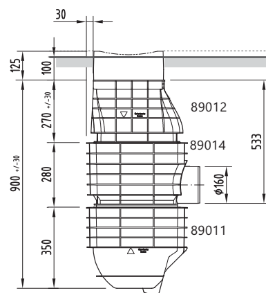
500 x 500 iszapfogós akna
