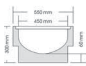
2a / alsórész Súly: 86 kg
