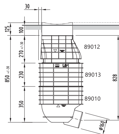
500 x 500 magas akna
