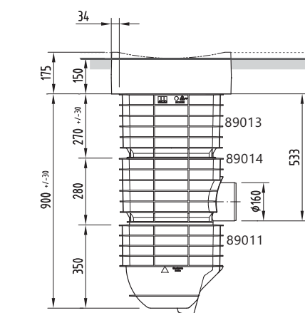
500 x 500 iszapfogós akna
