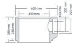
3a / közbenső elem Súly: 76 kg
