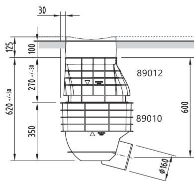
300 x 500 rövid akna
