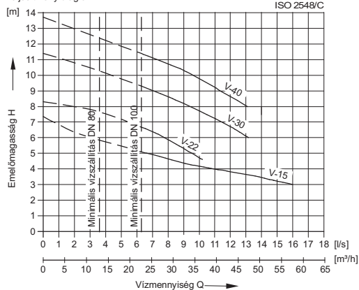
Teljesítmény diagram
