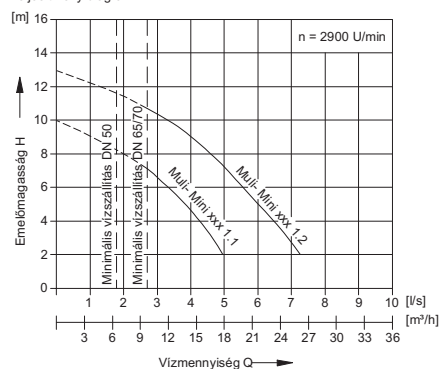
Teljesítmény diagram
