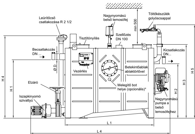
Lipurat-OAE (3. felszereltségi fok iszapkinyomó szivattyúval)
