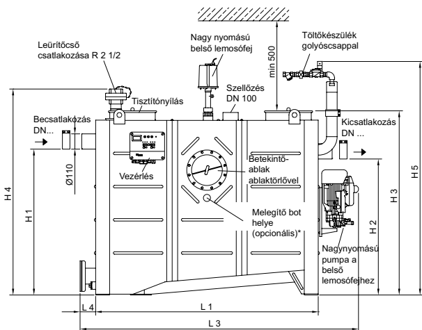
Lipurat-OA (3. felszereltségi fok)
