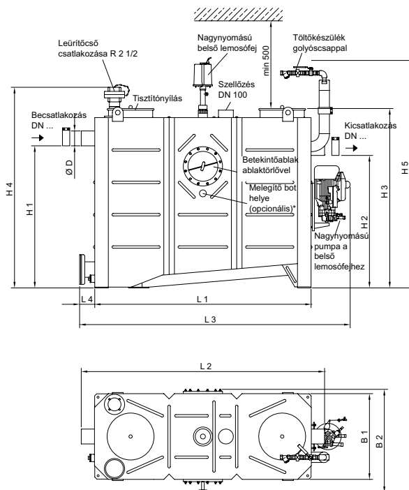
Lipurat-OS (2. felszereltségi fok)
